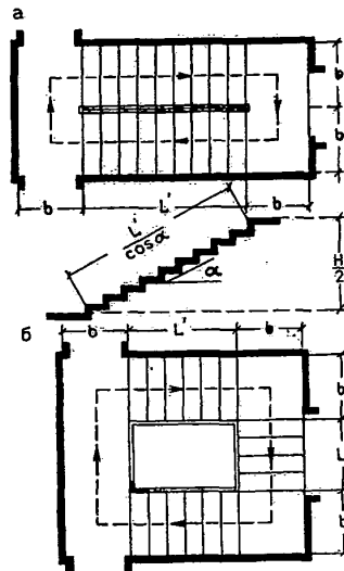
Рис. П5.1. Расчетная длина пути по лестнице:
