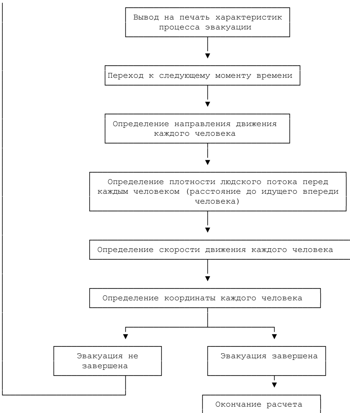
Рис. П3.2. Блок-схема определения расчетного времени эвакуации людей из здания
