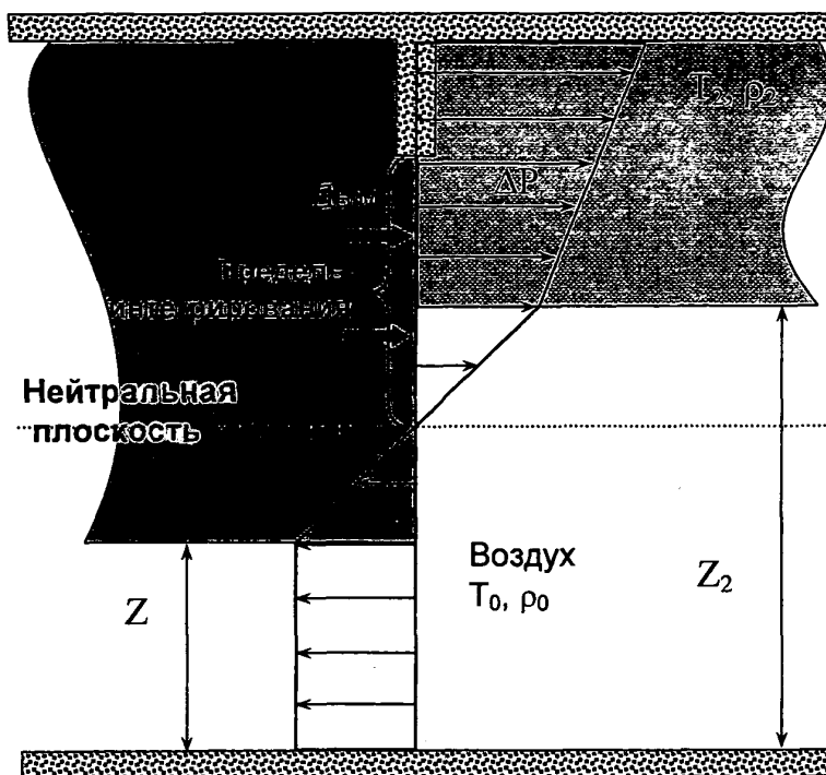
Рис. П6.1. Массопотоки через проем
