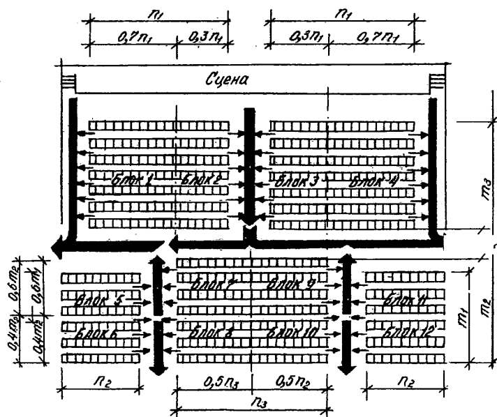
Рис. П5.3. Маршрутизация движения людских потоков при эвакуации из зрительных залов с боковыми (продольными) проходами
